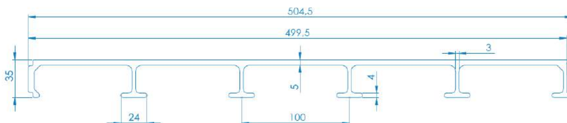
figuur 5: Geometrie plank 500.35
